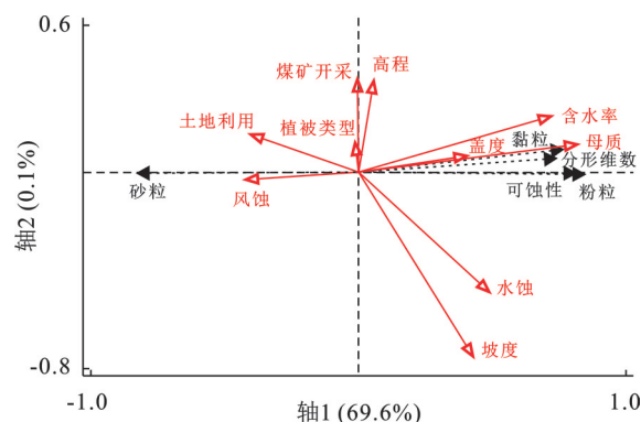
图4 研究区土壤粒径和K值与环境因子关系
